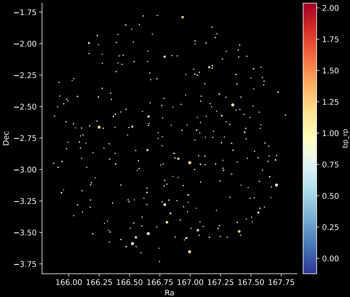
GALAH DR4 Field: [722] Stars: 291
