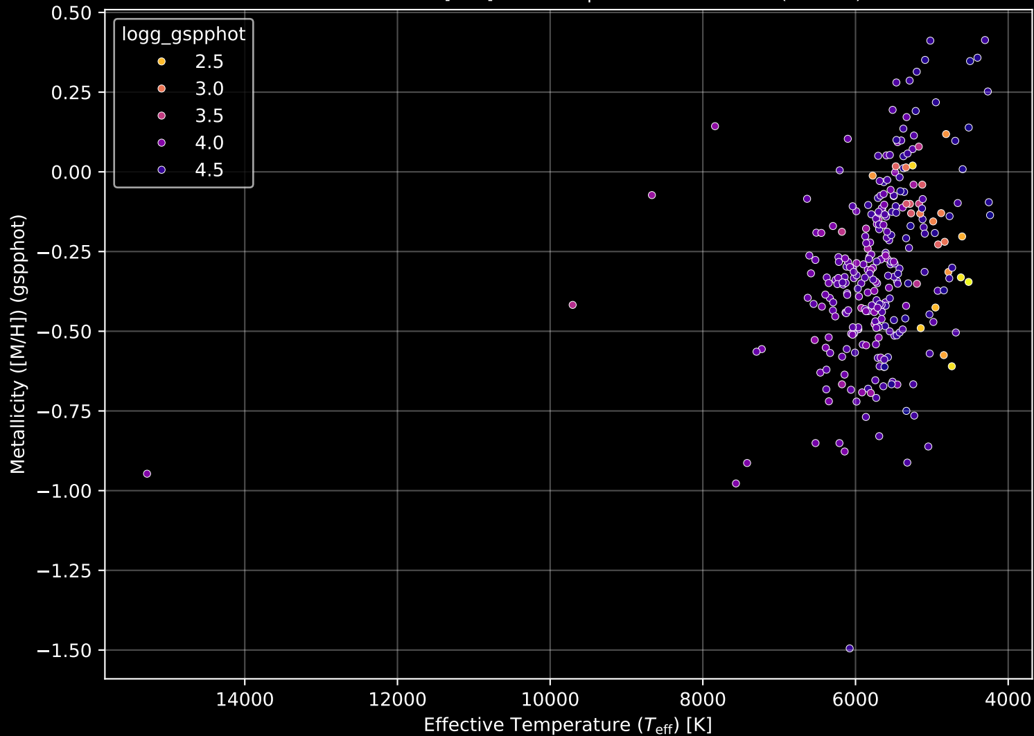
GALAH DR4 Field: [722] Stellar Population Parameters (n= 291)
